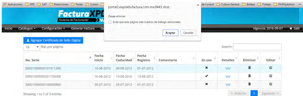
Imagen 4. Eliminar CSD
